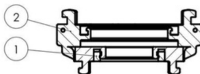
Corte A-A
